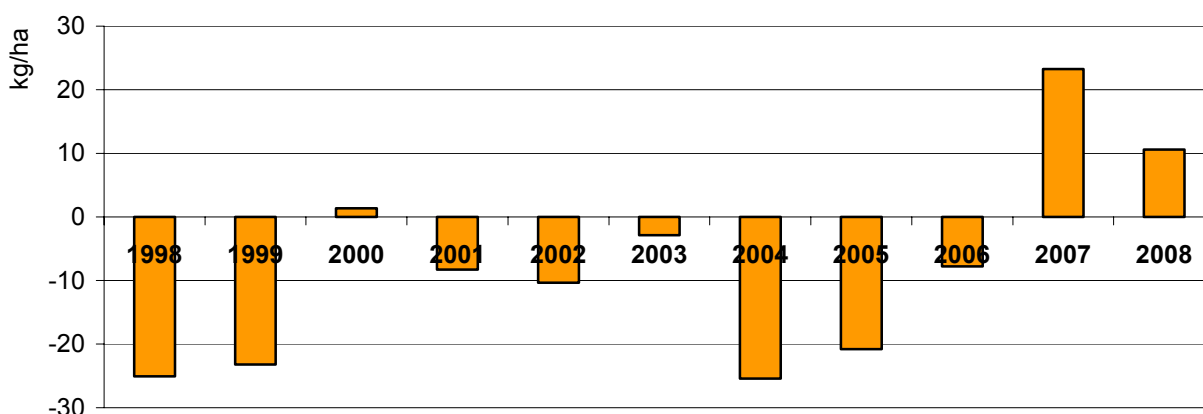
Obr. 9: Celková bilancia dusíka v poľnohospodárskych pôdach SR (kg/ha)
