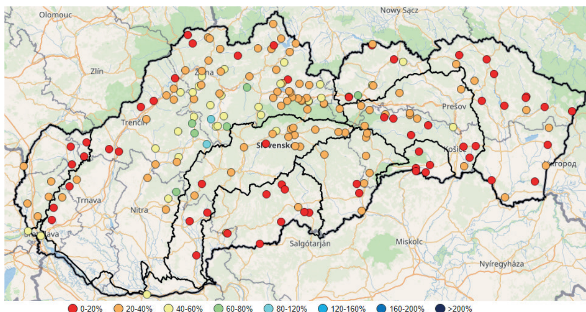
Mapa 022 | Situácia priemernej mesačnej vodnosti v SR – júl 2022 (operatívne údaje)
