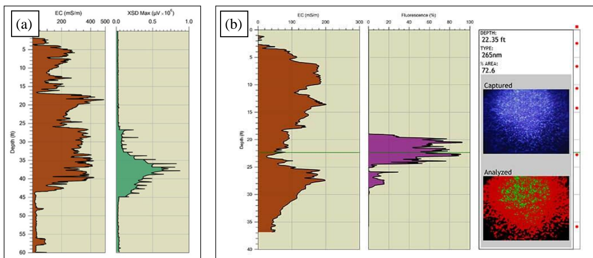
Obrázok 15. Príklad výstupu z merania vodivosti ( EC ) a koncentrácie prchavých uhl'ovodíkov ( XSD ) s integrovanou MIP sondou (a) a ukážka výstupu merania vodivosti ( EC ) a prítomnosti ľahkých uhl'ovodíkov fluorescenčnou metódou ( Fluorescence ) s integrovanou OIP sondou (b)
